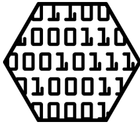
Infrastructure-as-a-Service
