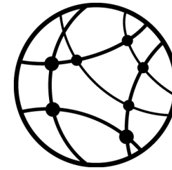
ISV
